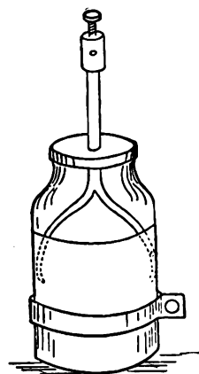
FIG. 2.—LEYDEN JAR
