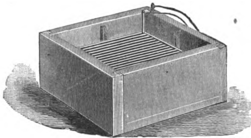
FIG. 23. TRAY CELL.
