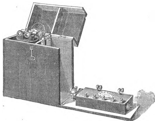
FIG. 13.—Small Faradic Apparatus. (Kidder.)
