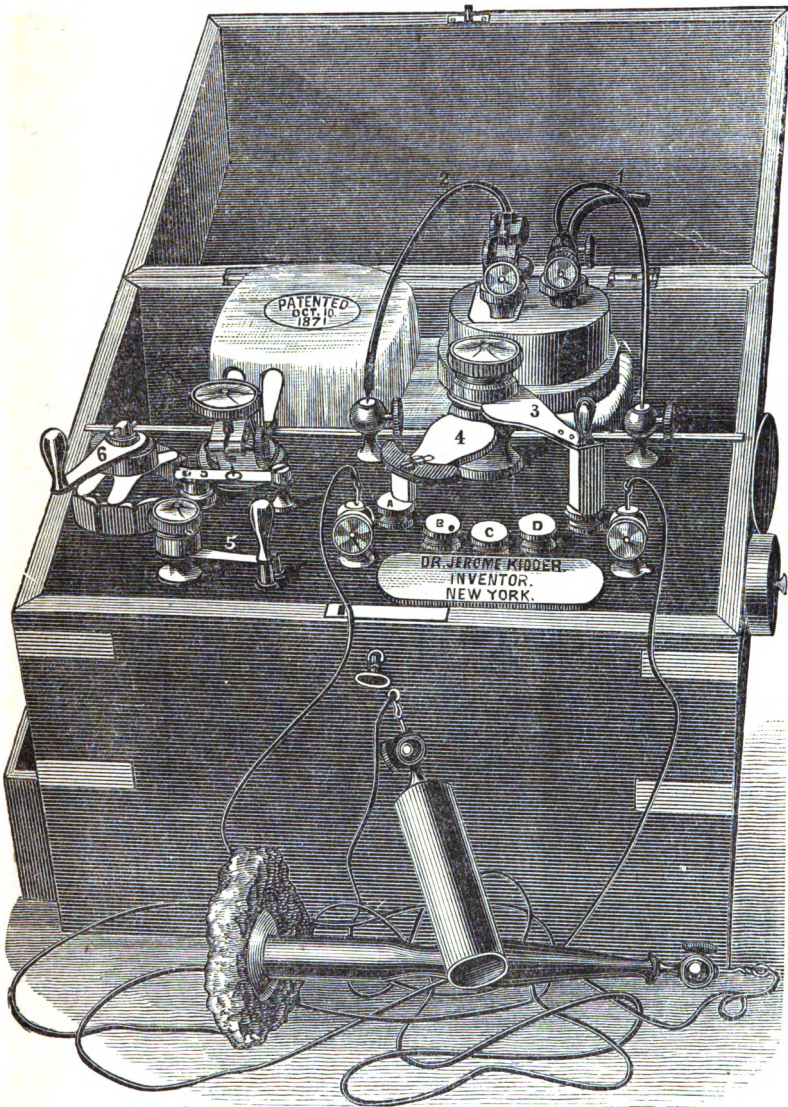
FIG. 12.—Faradic Apparatus. (Kidder.)
