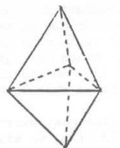
CALCITE CRYSTAL
